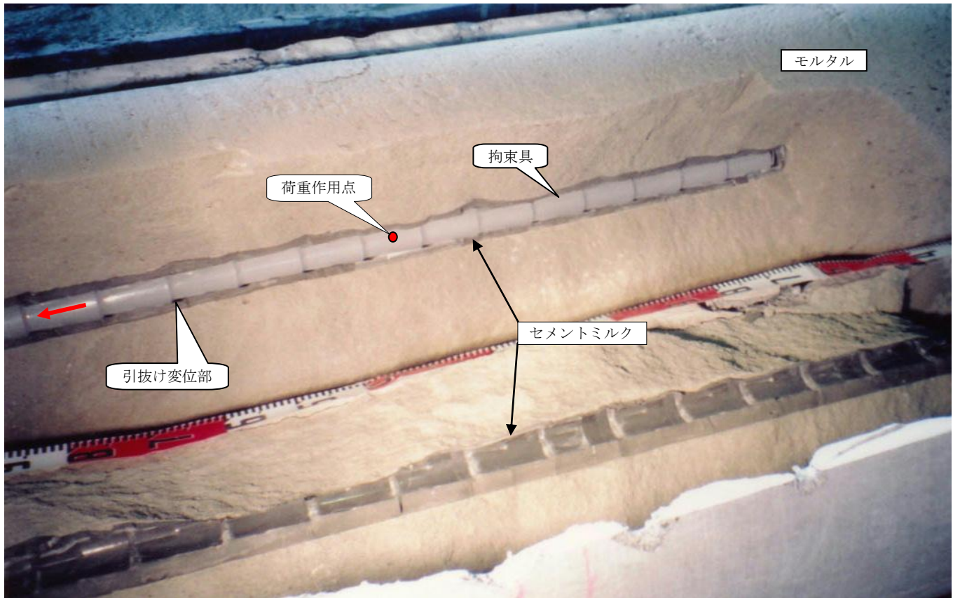
アンカー一体拘束具（くさび）定着状況
