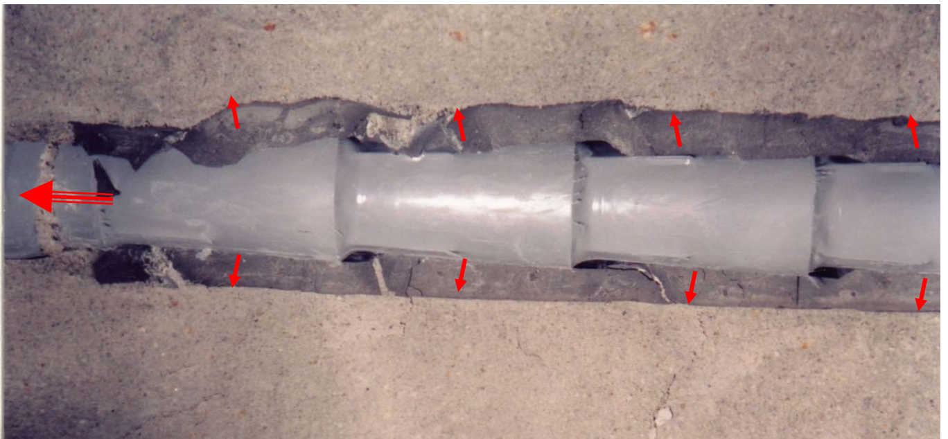
拘束具作動状況（超過荷重時）
