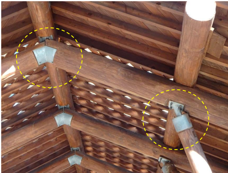
伝統的な木組み工法から、 金具を用いた在来工法に
