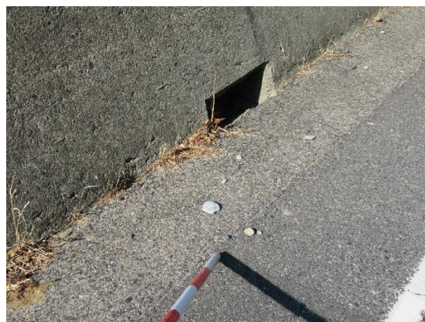
護岸：排水口を通して道路面まで打ち上げられた小石
