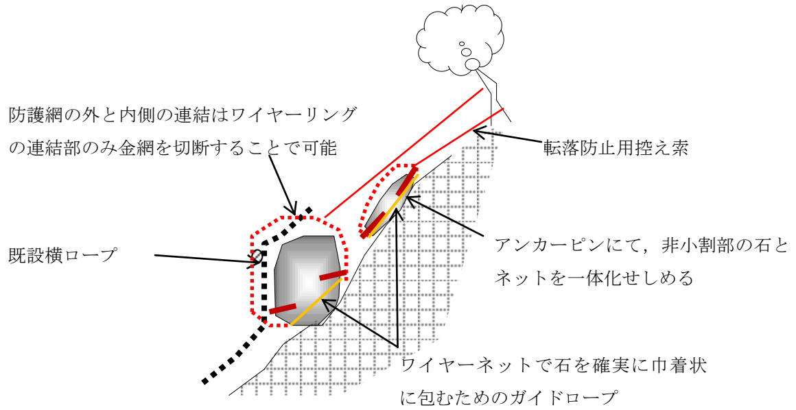
図-3 施工断面図
