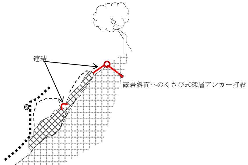
図-6 小割後の状態とアンカーによる固定
