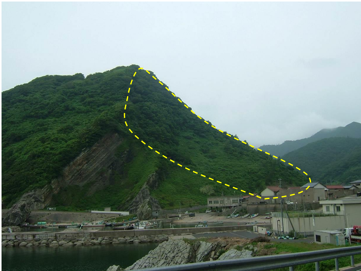
○受け盤のすべり（砂岩・泥岩）
