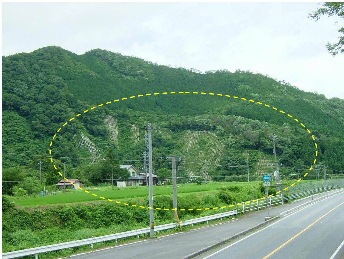
○法枠を基礎とした岩盤緑化（14年経過、鳥取西部地震）
